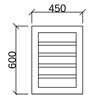
VENTILATOR - V2
