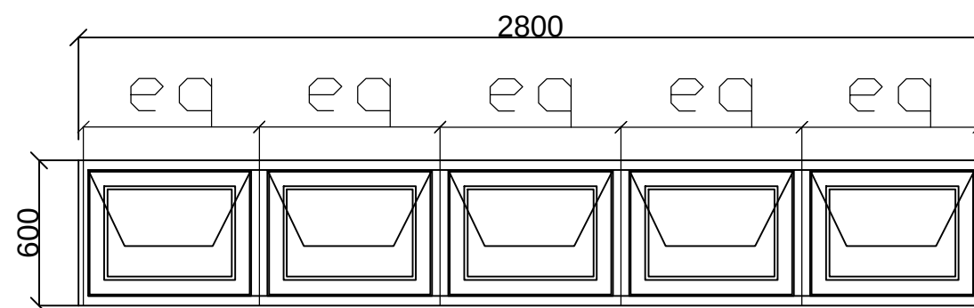
VENTILATOR TYPE-V/V1
